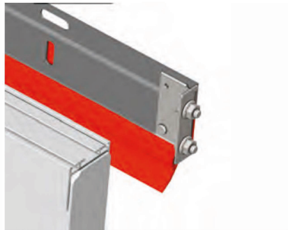
Profil support joint d'étanchéité en linteau
