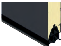
Joint bas à triple lèvre, isolation et étanchéité parfaite au sol
