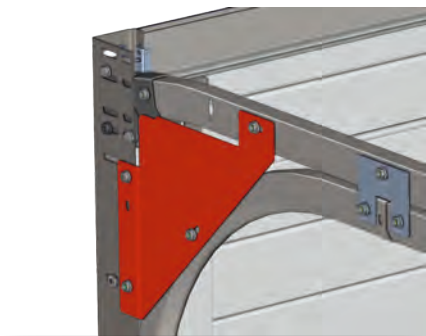
Plaque renfort sur courbes
