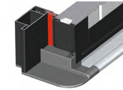
Joint d'étanchéité tubulaire EPDM côté ouverture
