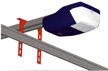
Motorisation BFT Tiziano et système easyfixe
