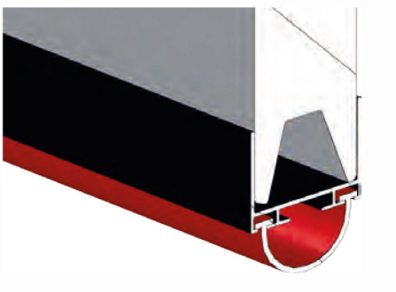
Joint à bulle EPDM sur panneau bas
