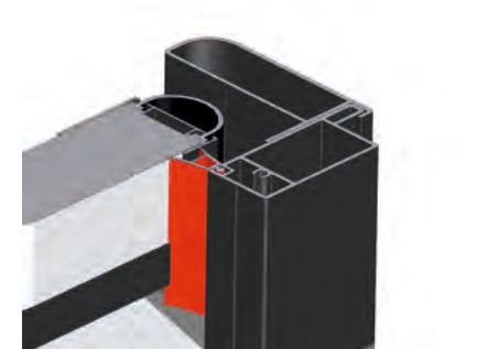
Joint tubulaire à lèvre EPDM côté fermeture
