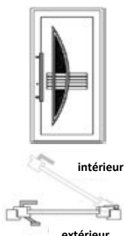
Porte DIN gauche ouvrant vers l'intérieur : Panneau de porte DIN gauche
